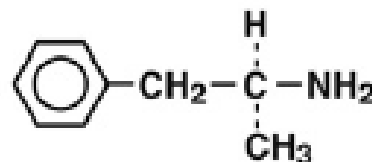
D-Amphetamine
